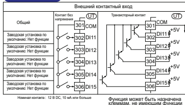
301-306 Область клемм E1
