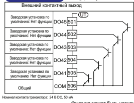
501-506 Область клемм E4
